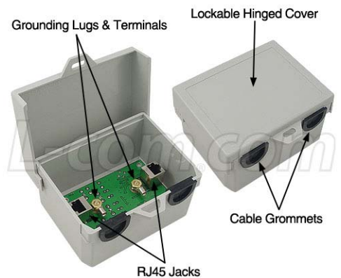
Model: AL-CAT5EJW24
